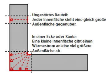
Das Prinzip der geometrischen Wärmebrücke in der Kante Außenwand. Die Pfeile symbolisieren den Wärmestrom.
